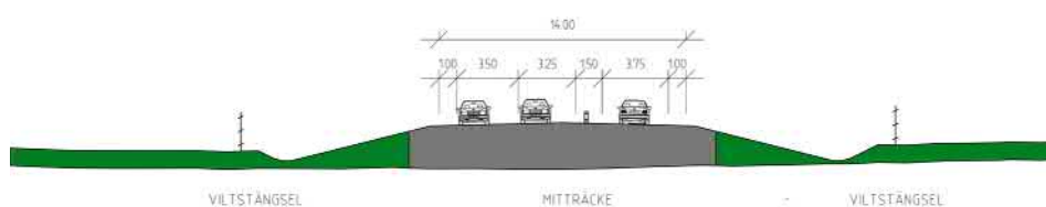
Figur 12 Vägen ligger på bank med långa, flacka slänter 1:3, ner till vägdikena.
