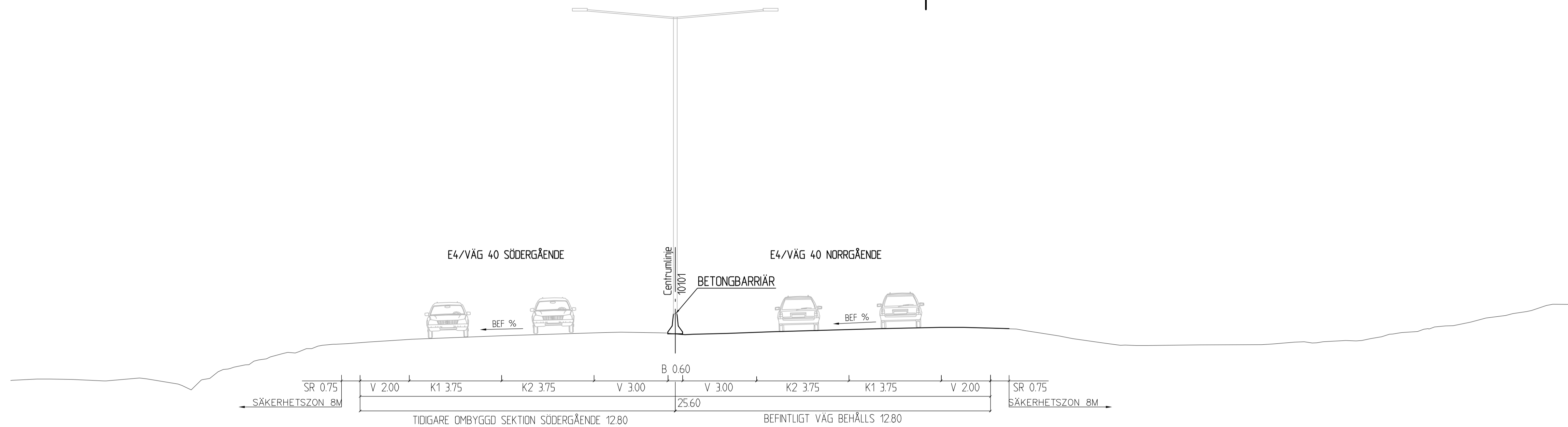
TYPSEKTION 07 E4 (MITTFÖR TRAFIKPLATS RYHOV) VÄGLINJE 10101, 3/250
