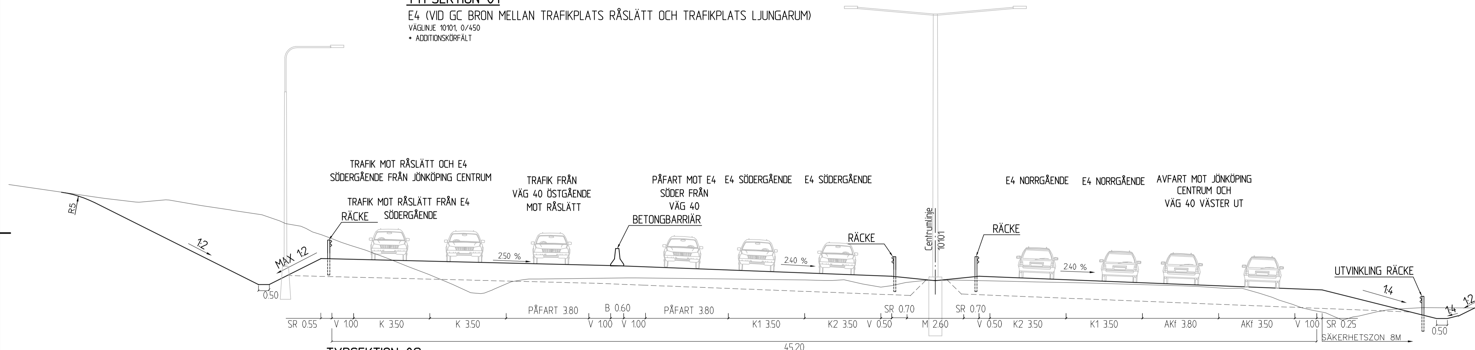
TYPSEKTION 02 E4 (I HÖJD MED LJUNGARUMSSKOLAN MELLAN TRAFIKPLATS RÅSLÄTT OCH TRAFIKPLATS LJUNGARUM) VÄGLINJE 10101, 0/700
