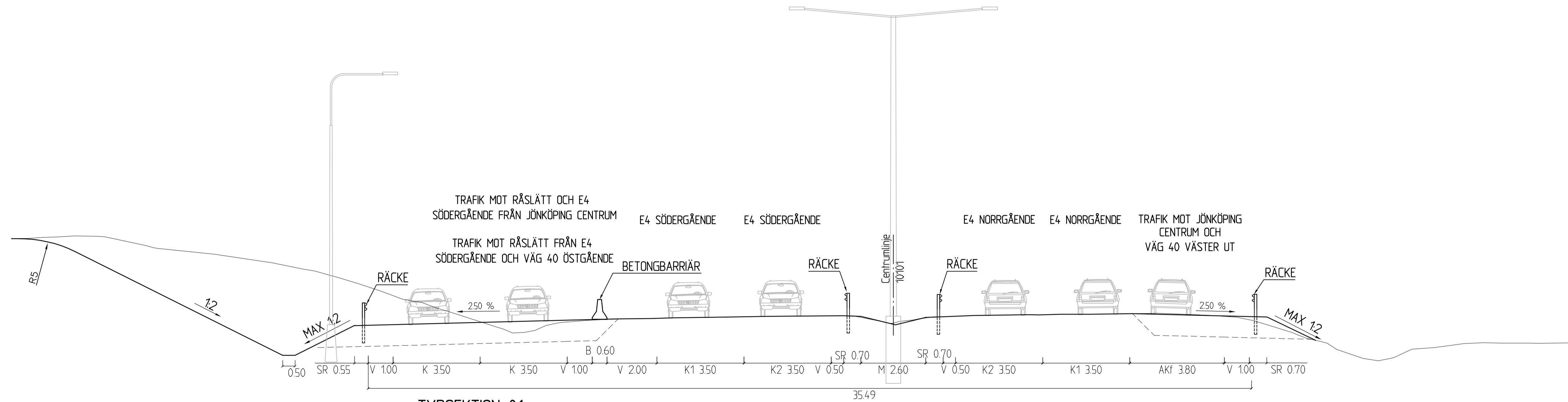
TYPSEKTION 01 E4 (VID GC BRON MELLAN TRAFIKPLATS RÅSLÄTT OCH TRAFIKPLATS LJUNGARUM) VÄGLINJE 10101, 0/450 • ADDITIONSKÖRFÄLT
