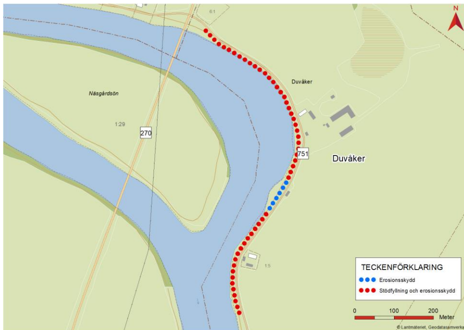
Figur 10 Aktuell sträcka i Duvåker för stödfyllning och erosionskydd.
