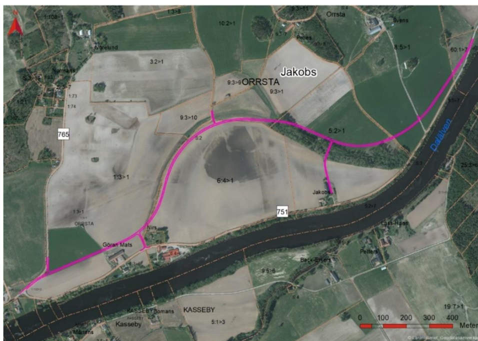
Figur 19 Förordat riskreducerande åtgärd i Jakobs. Illustrerad med föreslagna förändringar utifrån alternativ Röd.
