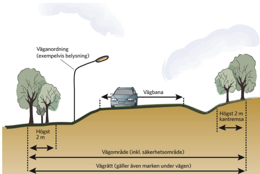
Figur 24. Illustration över vägrätt, vägområde, väganordning och vägbanan. Källa: Trafikverket.
