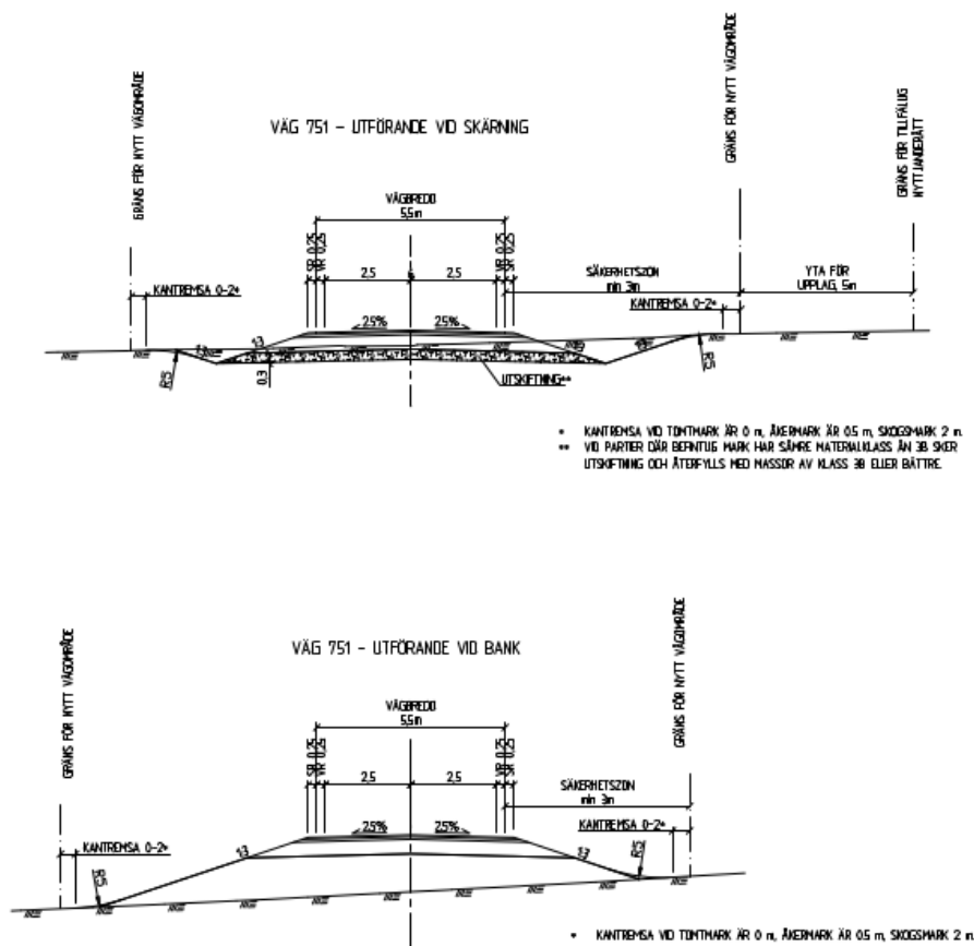
Figur 21. Principutformning av väg.
