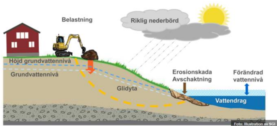
Figur 3. Bildförklaring av orsak till skred. Källa: SGI.
