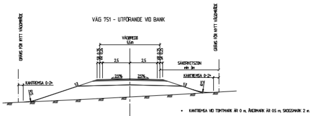
Figur 22. Principutförning av väg.
