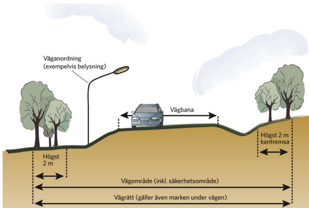
Figur 24. Illustration över vägområde, vägrätt, väganordning och vägbana. Källa: Trafikverket.
