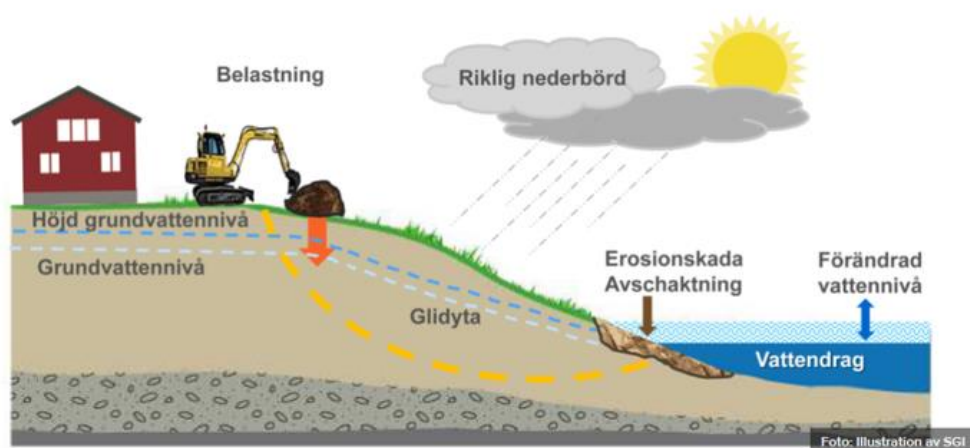
Figur 3. Bildförklaring av orsak till skred. Källa: SGI.
