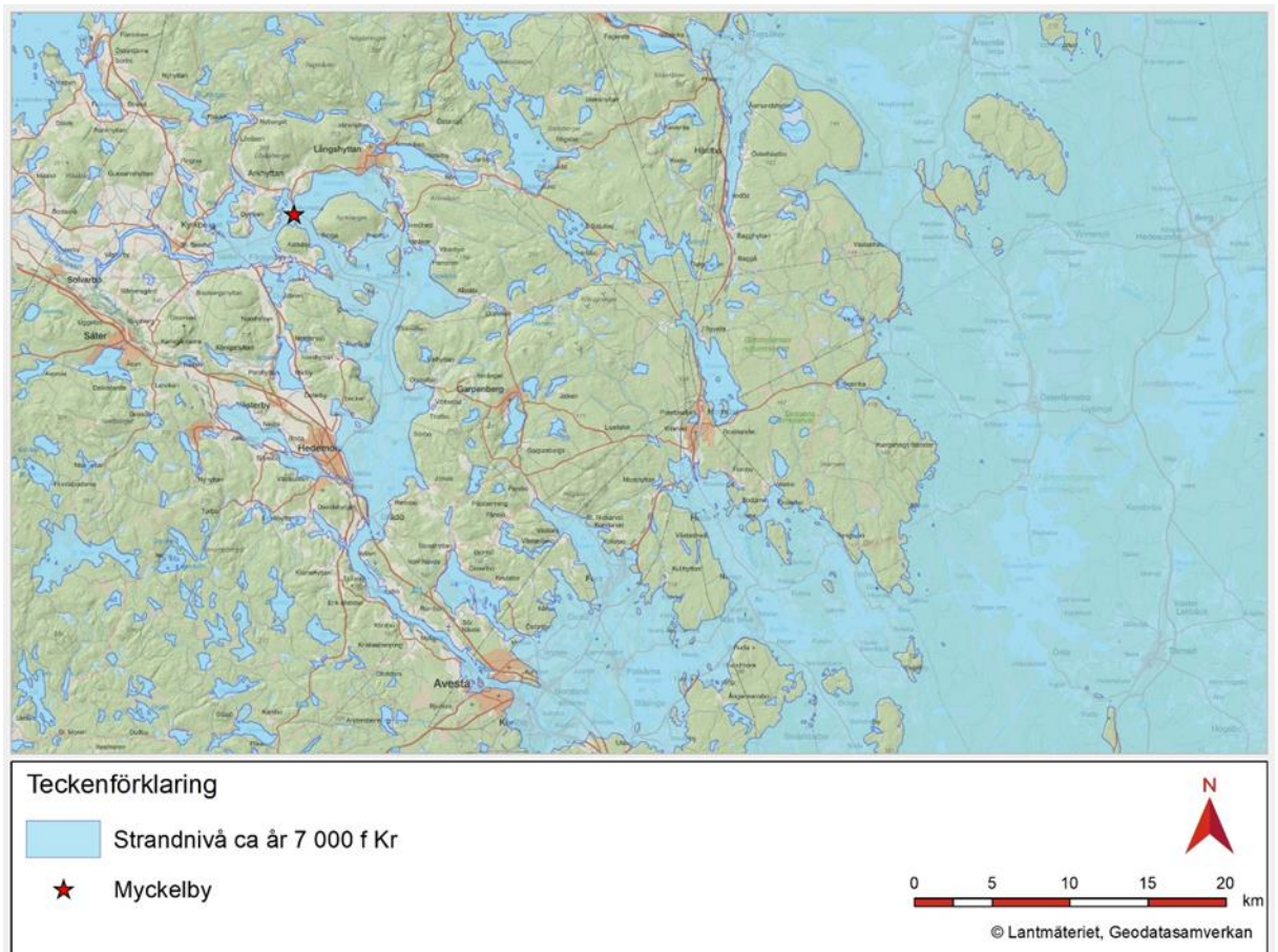
Figur 14. Strandlinjen omkring 7000 f Kr. De flacka områdena var vid denna tidpunkt en större havsvik.
