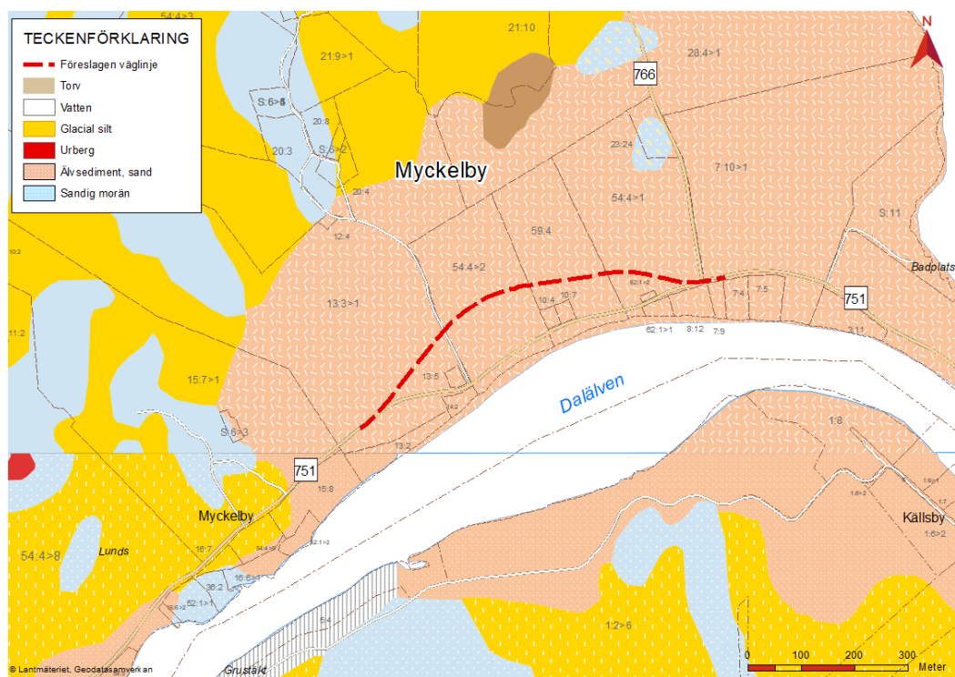
Figur 10 .Jordartskarta från Sveriges geologiska undersökning (SGU).
