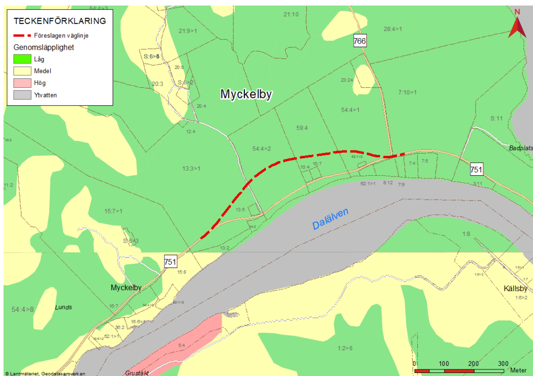
Figur 9. Genomsläpplighetskartan från SGU indikerar att området har låg genomsläpplighet.
