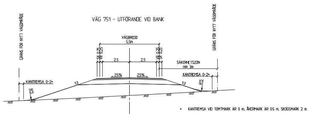
Figur 24. Principutförning av väg.
