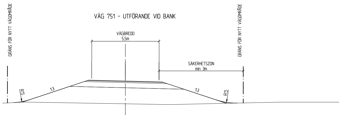
Figur 13. Typsektion Jakobs
