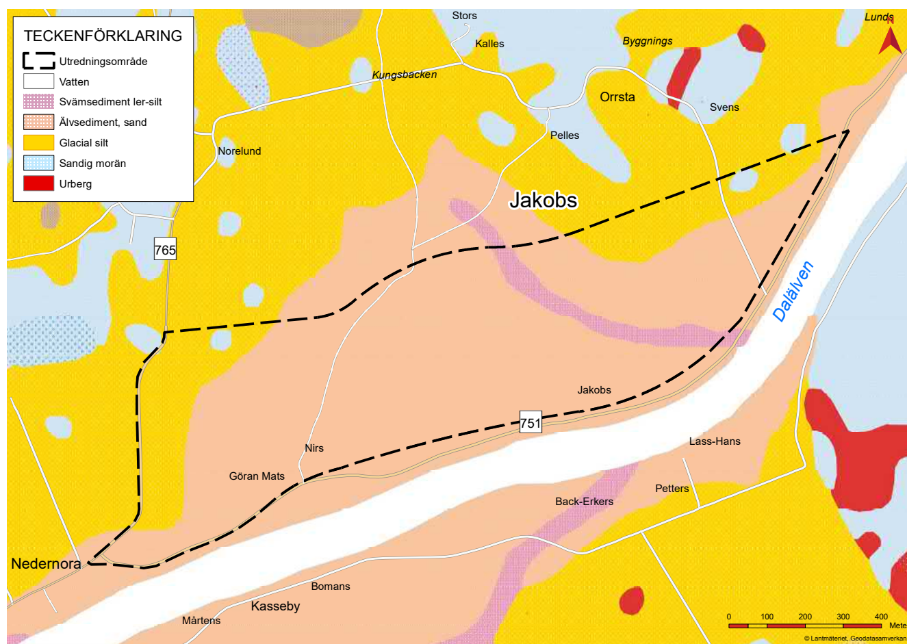
Figur 4. Jordartskartan.
