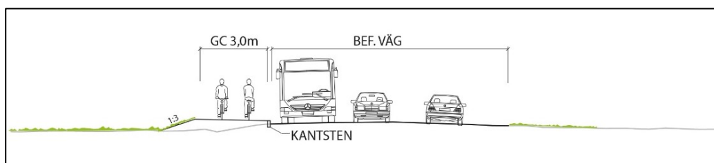
Figur 8. Sektion 0/950 som visar hur gång- och cykelvägen passerar busshållplatsen Eriksborg, sedd österifrån. Gång- och cykelvägen är åtskild från körbanan med en kantsten.
